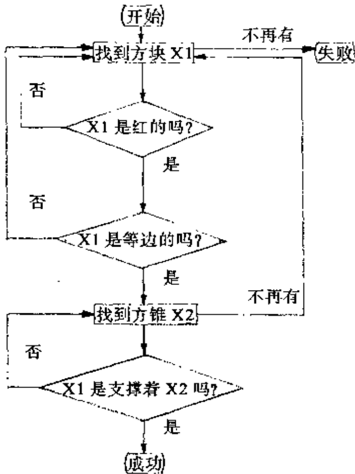
图 118. 对“一个支撑着方锥的红立方体”的过程化表示。[引自罗杰·尚克和肯尼恩·科尔比,《思维的计算机模型和语言》,172页。]
