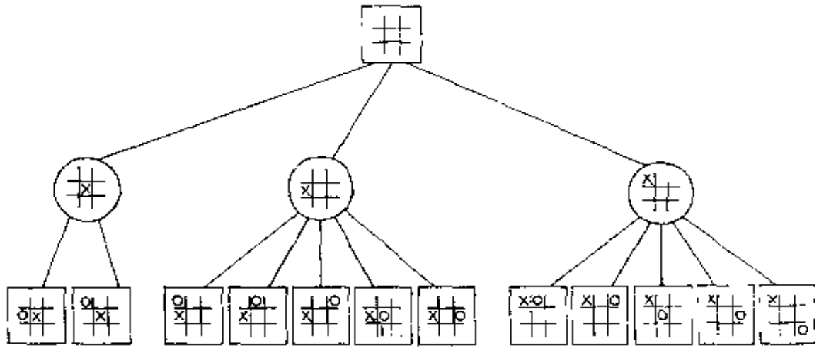
图 38. 三子棋开始两步的超前搜索树。
