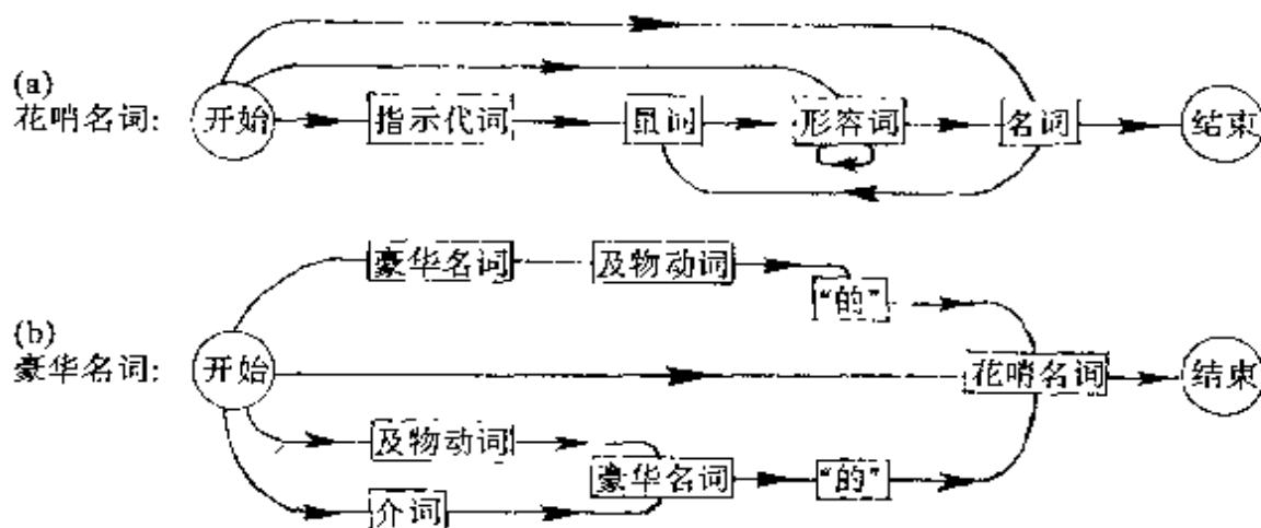
图 27. 花哨名词与豪华名词的递归迁移网。
