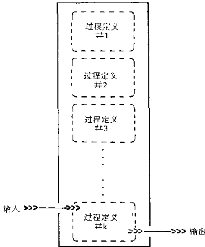
图72. 一个待调用的 BlooP 程序的结构。由于这个程序是自足的,每个过程定义中只能调用定义在它前面的过程。
