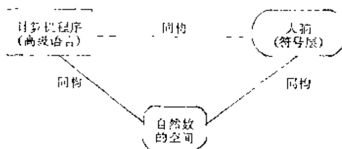
图 106. 自然数的性质能在人类大脑和计算机程序中得到反映。这两个不同的描述因而能在一个适当的抽象层次上彼此对应。
