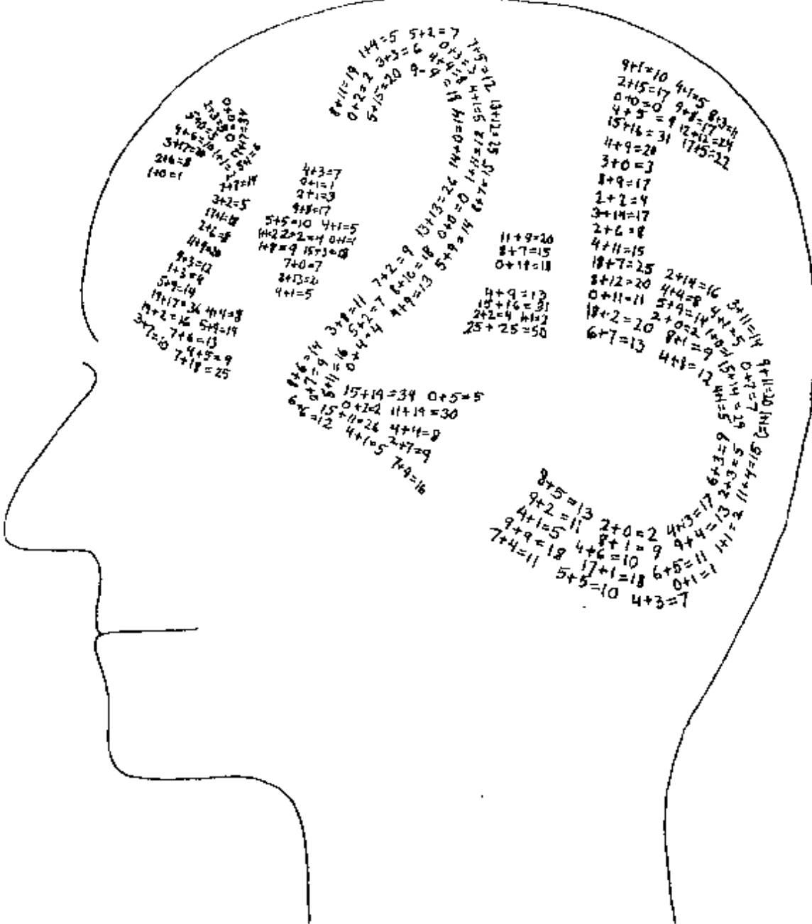
图 109. 大脑是理性的,而心智则可能不是。[作者绘]
