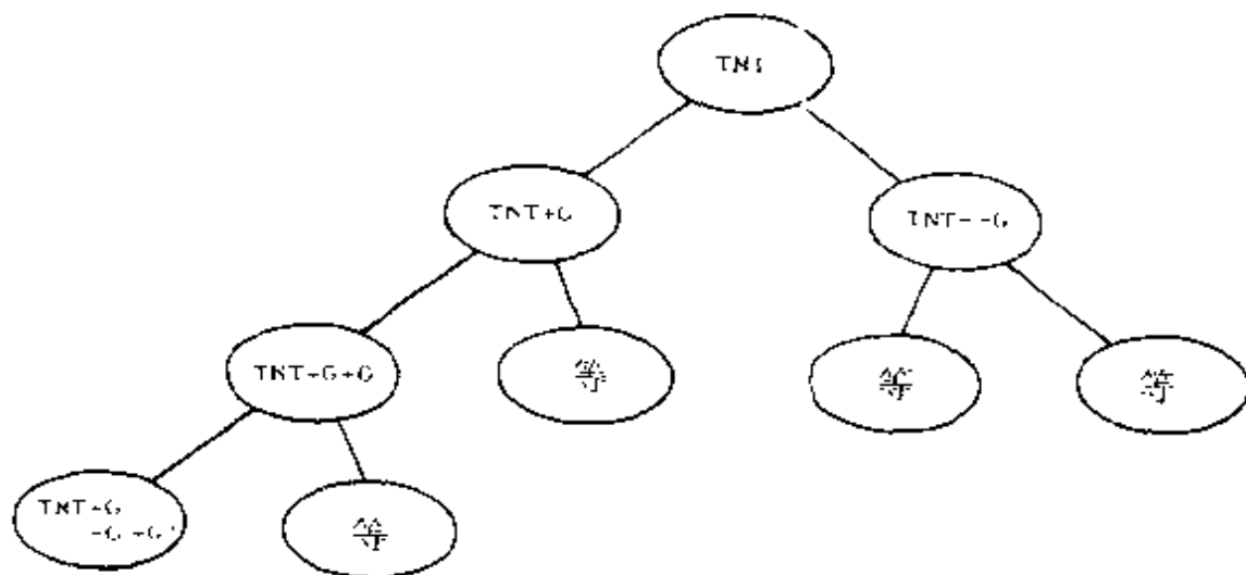
图 75. TNT 的“多重分叉现象”。TNT 的每个扩充都有它自己的哥德尔句子,可以把这个句子或其否定添加进去,使得从 TNT 的每个扩充都生出一对进一步的扩充。这是一个直到无穷的过程。
