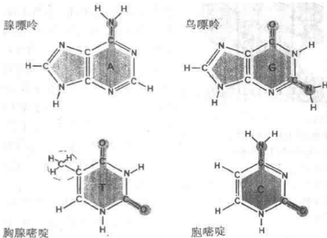
图 91. DNA 的四种基：腺嘌呤，鸟嘌呤，胞嘧啶，胸腺嘧啶。[摘自哈那瓦尔特和海因斯 [Hanawalt; Haynes], 《生命的化学基础》[The Chemical Basis of Life], 旧金山; W. H. Freeman, 1973 年版, 第 142 页。]
