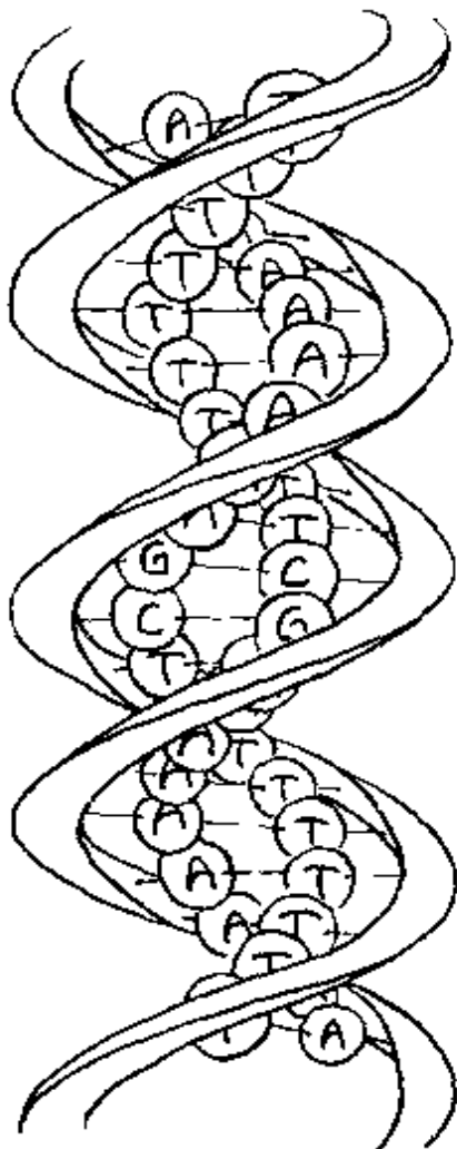
图 43. 这里是螃蟹的一种基因中的一小段，它们一圈圈地缠绕着。当两股 DNA 链被拆开并且并排铺开时，它们读起来是这样的：
