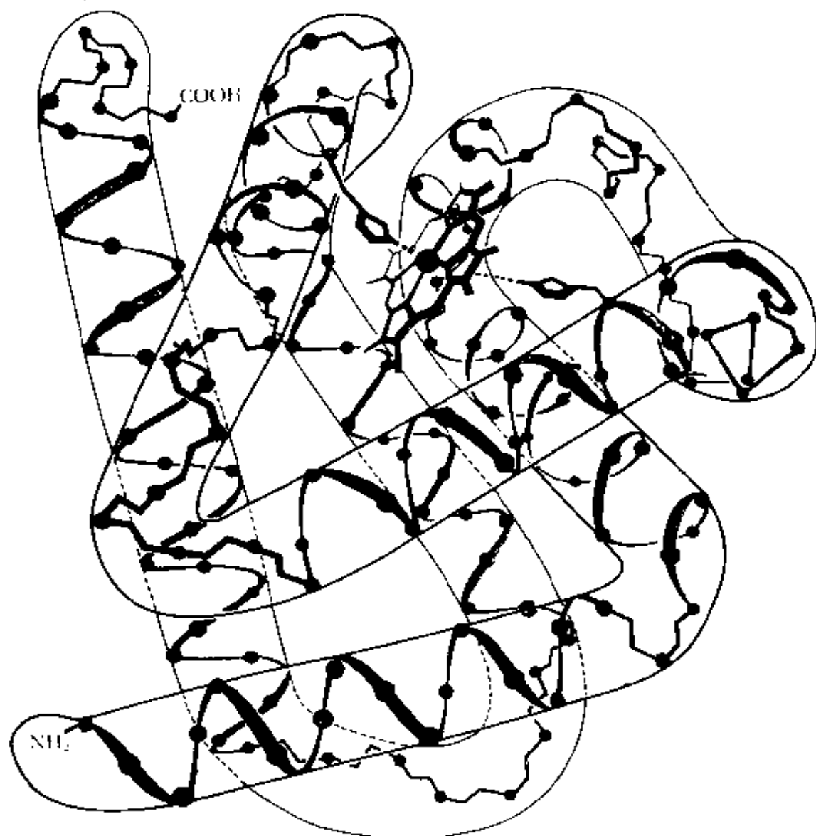
图 95. 从一些高分辨率的 X 光资料推断出的肌红蛋白的结构。大尺寸的“扭曲管道”形状是三级结构,内部的细螺旋——“阿尔法螺旋”——是二级结构。[选自莱宁格尔,《生物化学》。]
