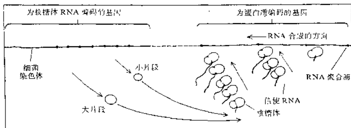
图 98. 这里是一个更为复杂的图示,不只一个而是有若干个 mRNA 串,它们全都转录自同一个 DNA 串,并受到多核糖体作用,其结果是一个二排分子卡农。「选自哈那瓦尔特和海因斯,《生命的化学基础》,第 271 页。」
