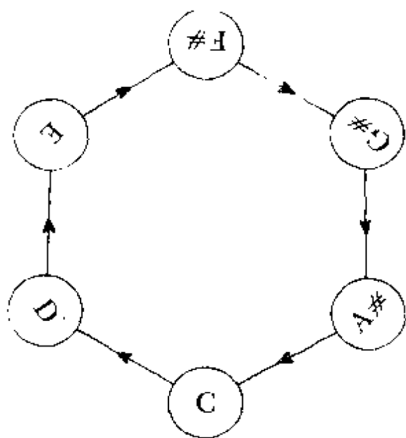
图 147. 巴赫的“无穷升高的卡农”的六角形示意图。在使用谢泼德音调的条件下，它形成了一个不折不扣的闭合循环。
