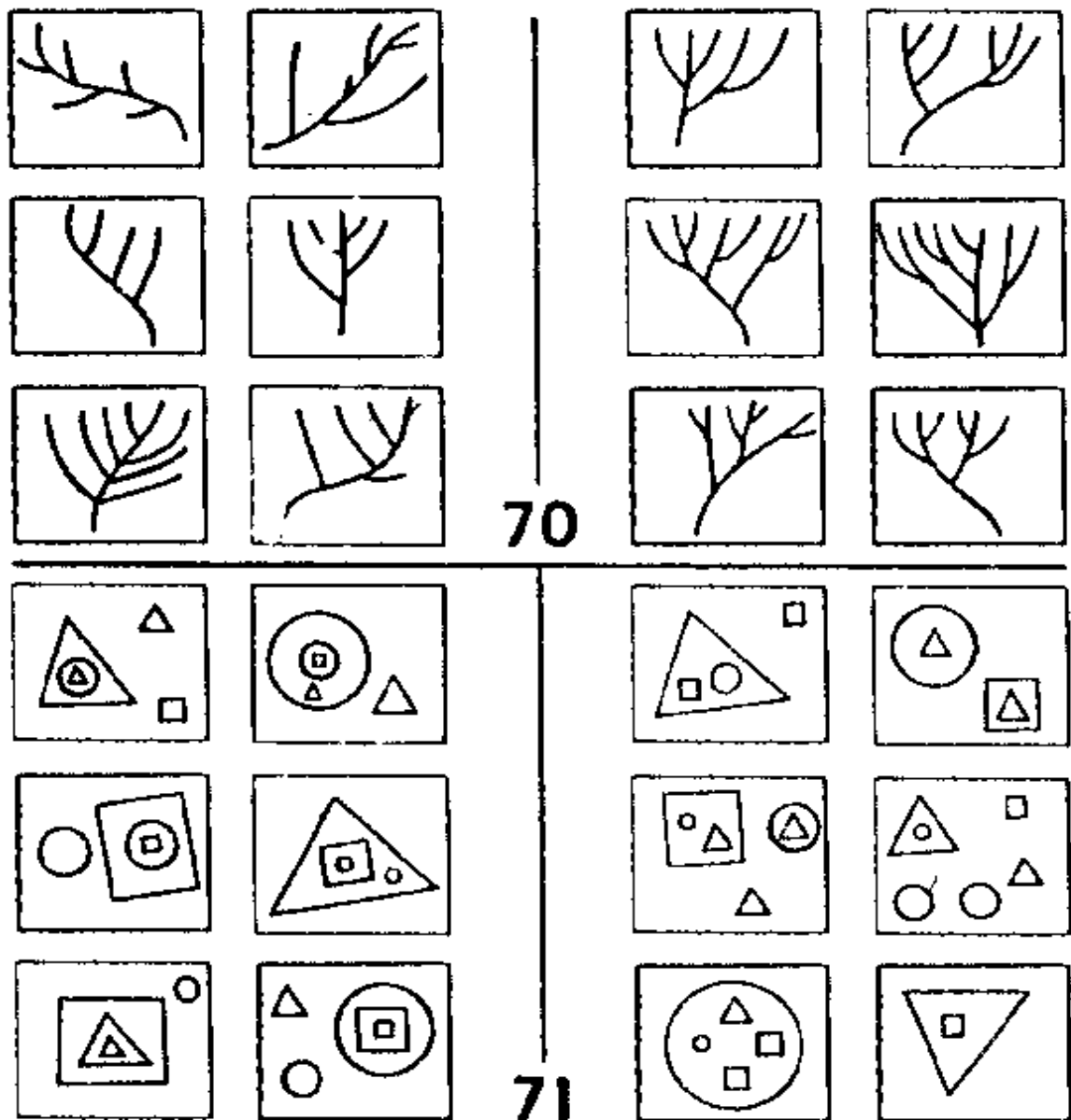
图 130. 邦加德问题 70~71 号。[摘自莫·邦加德,《模式识别》。]
