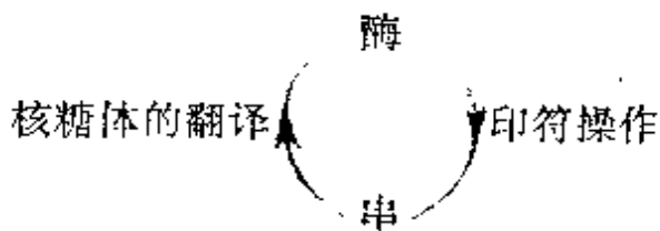
图 90. “印符遗传学的中心法则”: “缠结的层次结构”的一个例子。
