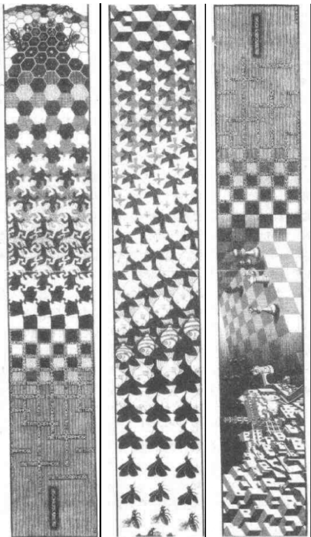
图 8. 变形 I, 艾舍尔作(木刻, 19.5 × 400 厘米, 1939--1940)。
