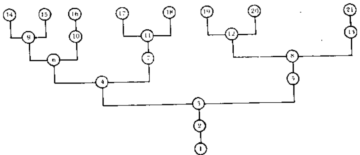
图 30. 图案 G, 进一步地扩展了, 并为结点标了数字。
