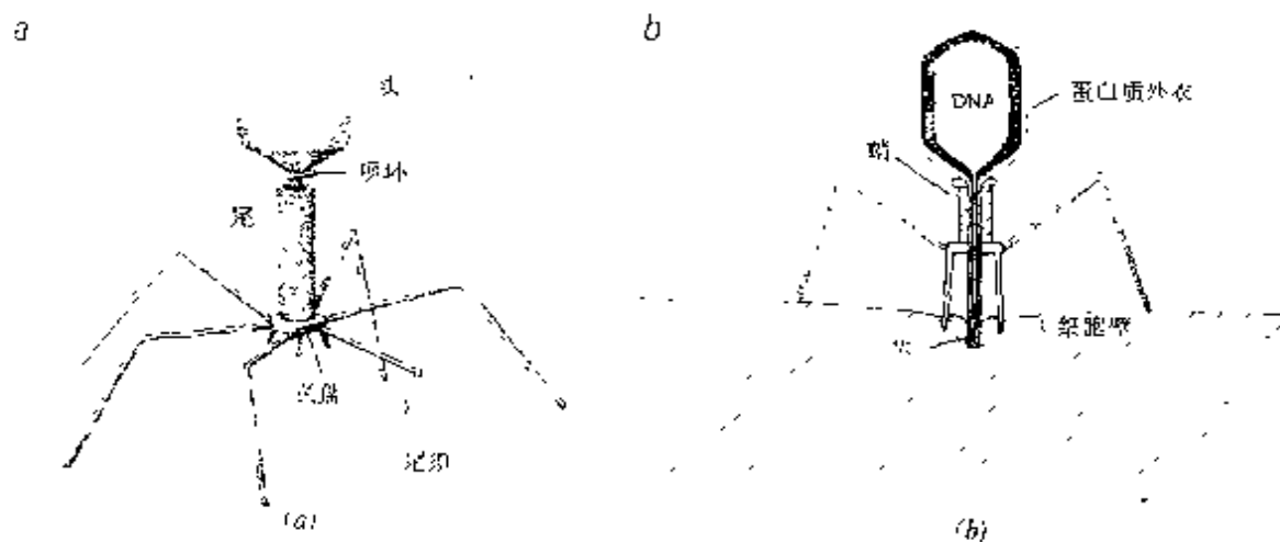
图 101. T4 细菌病毒是一个蛋白质聚合体(a)。它的“头”是形如一种具有三十面的扁长的正十二面体的蛋白质膜，里面充满了 DNA，头通过一个颈与尾部相连。尾部是包在一个可收缩的鞘内的空心芯子，安在四周有六条须根、下面有若干钉子的底盘上。钉子和须根使病毒牢牢地粘在细菌的细胞壁上(b)。鞘的收缩使芯子穿透细胞壁，病毒的 DNA 进入细胞。〔选自哈那瓦尔特和海因斯，《生命的化学基础》，第 230 页。〕
