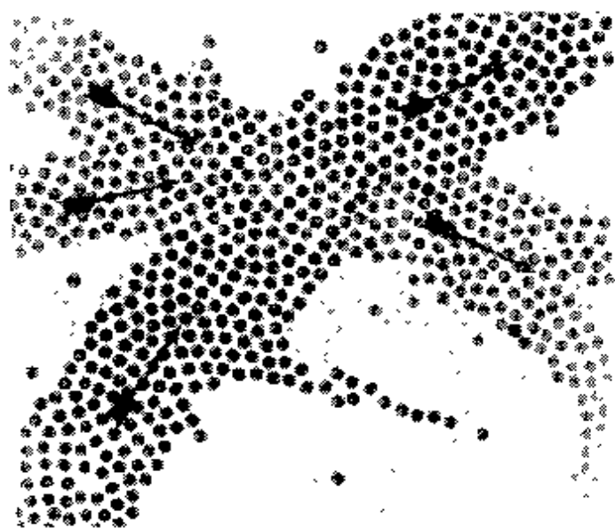
图 68. 在这张示意图中，假设神经原成点状分布在一个平面上。两条互相交叉的神经通道用不同的灰度来表示。可能出现这样的情况：两个独立的“神经闪电”同时通过这两条通道，像池塘水面上的两个涟漪一样彼此穿过（见图 52）。这形象地说明了两个共享神经原的“活跃符号”是如何可能同时被激活的。[摘自约翰·西·艾克勒斯 [John C. Eccles]，《面对现实》[Facing Reality]，纽约：Springer Verlag, 1970 年版，第 21 页。]
