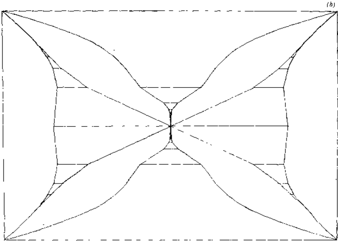
图 33. (b)能用递归替换构造 G 图的骨架。
