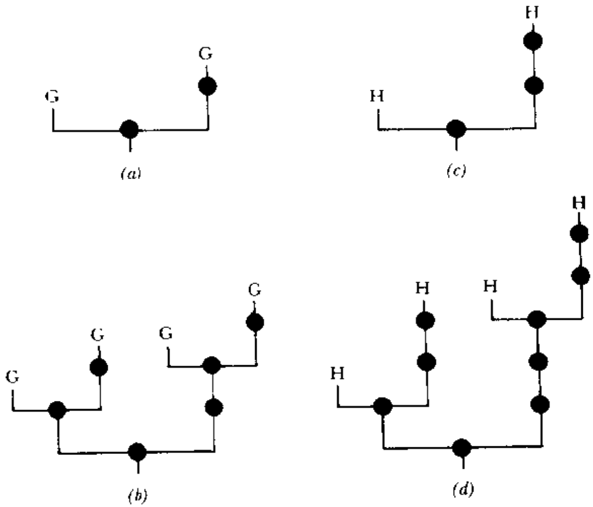
图 29. (a) 图案 G, 未扩展。 (c) 图案 H, 未扩展。 (b) 图案 G, 扩展一次。 (d) 图案 H, 扩展一次。
