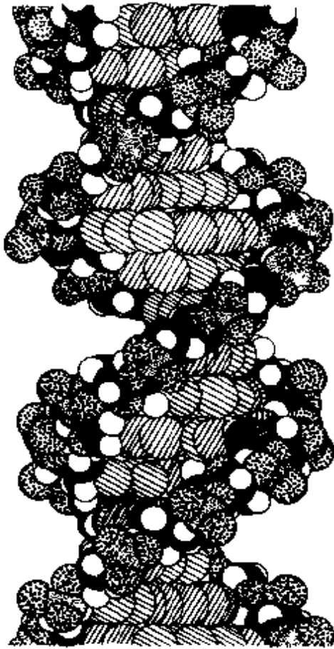
图 92. DNA 结构象一架梯子。边上两条由脱氧核糖和磷酸盐的单元交替组成，横档以特殊方式配对——A 配 T，G 配 C——的基形成，基之间分别由两个或三个氢键相互连接。[摘自哈那瓦尔特和海因斯，《生命的化学基础》，第 142 页。]
