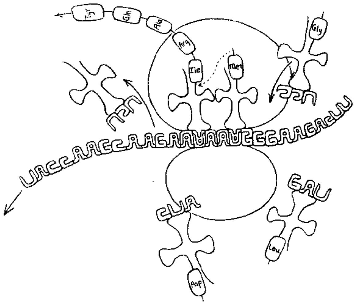
图 96. 一段 mRNA 通过核糖体。漂浮在附近的是些 tRNA 分子，它们带有能被核糖体抓来并加进正在生成的蛋白质中的氨基酸。遗传密码作为一个整体包含在 tRNA 分子内。要注意，基对 (A-U, C-G) 在图中由卡在一起的字型表示。[斯科特·凯姆绘]
