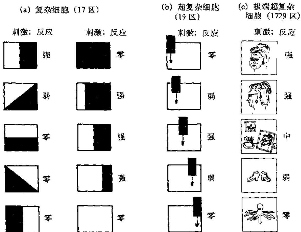
图 67. 某些神经原样本对模式的反应。
