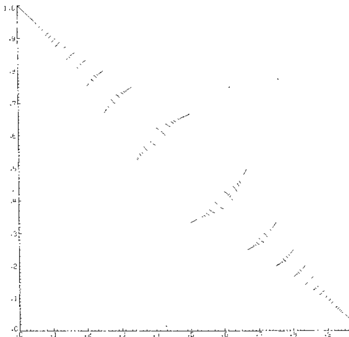
图 32. 函数 \text{INT}(x) 的图形。在 x 的每个有理数值处都是个跳跃性的不连续点。
