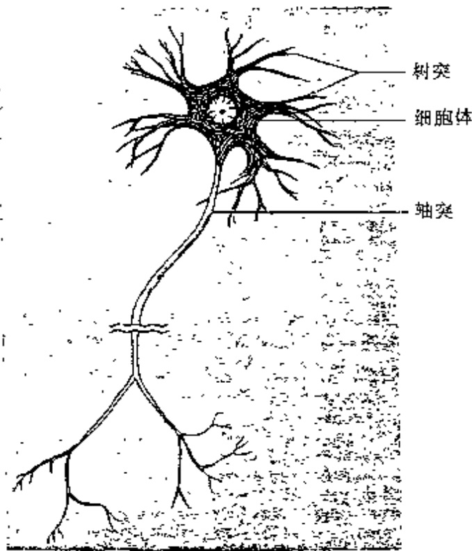
图 65. 神经原示意图[摘自伍尔德里奇 [D. Wooldridge], 《大脑的机制》[The Machinery of the Brain], 纽约: McGraw-Hill, 1963 年版, 第 6 页。]
