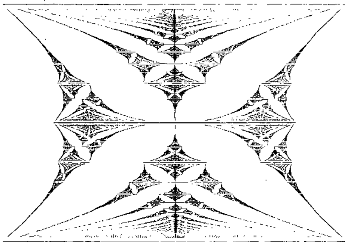
图 34. G 图:一个递归图形,显示了一个磁场中理想晶体里的电子的能量带。 \alpha 代表磁场强度,沿垂直方向从 0 到 1。能量是沿水平方向的。水平的线段是所允许的电子能量带。
