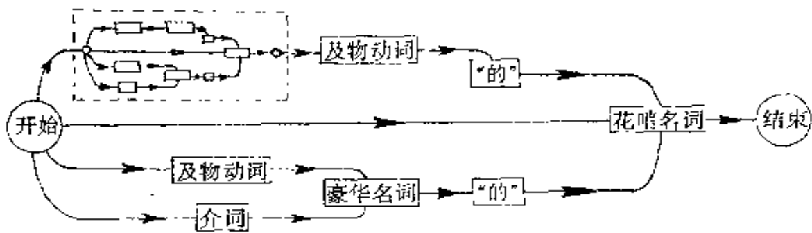
图 28. 豪华名词的 RTN, 其中有一个结点递归地扩展了。
